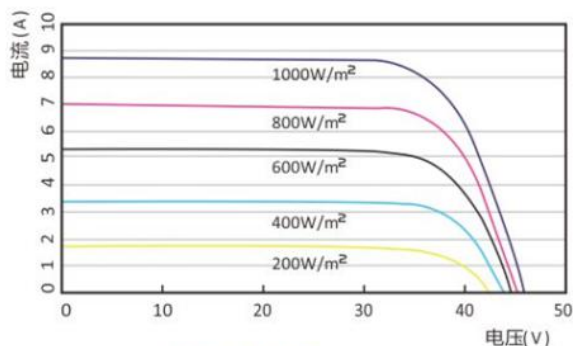
I-V 曲线
